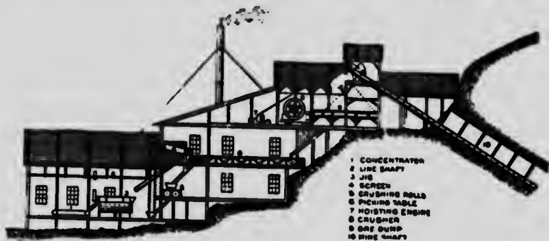
Fig. 1—Croquis montrant une coupe et élévation de l'une de fabrication mécanique et de concentration.
